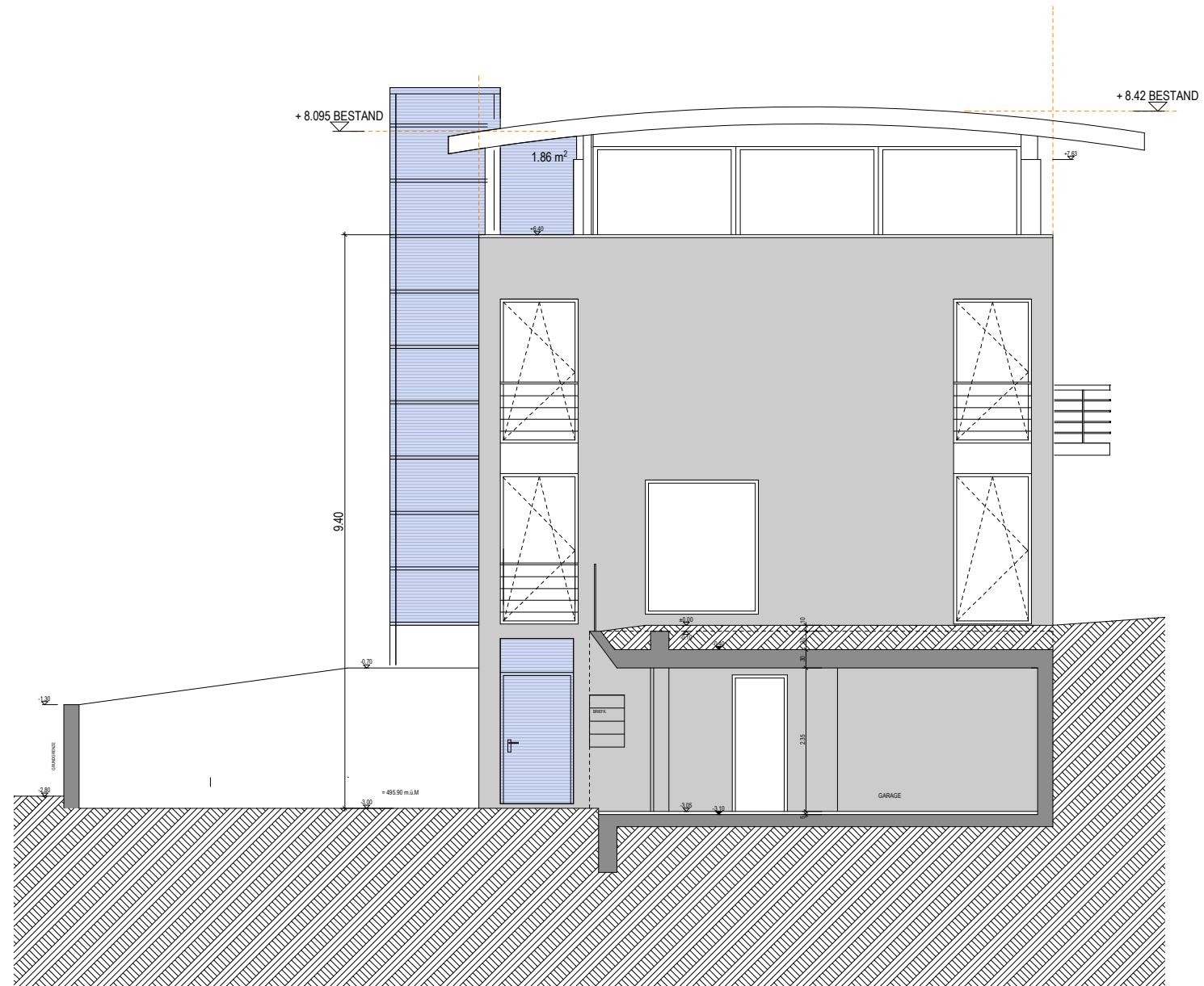
Ansicht Süd
