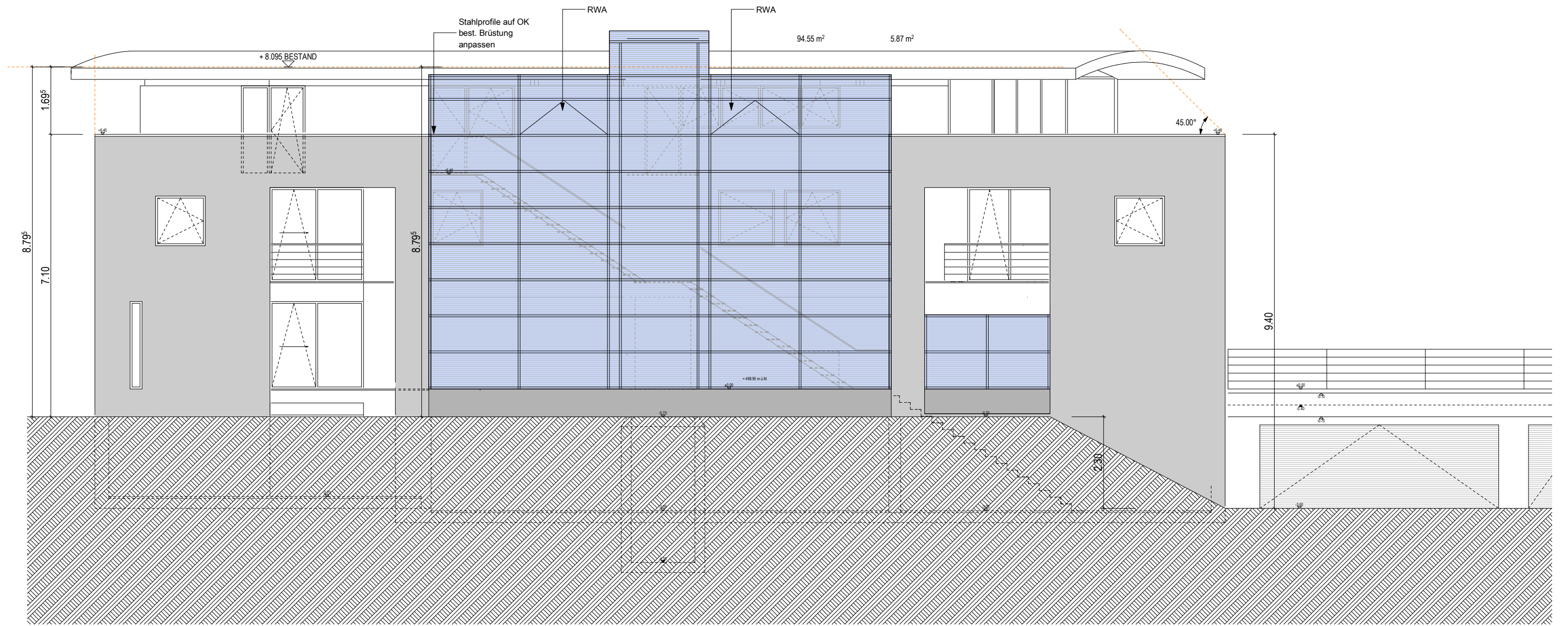
Ansicht West
