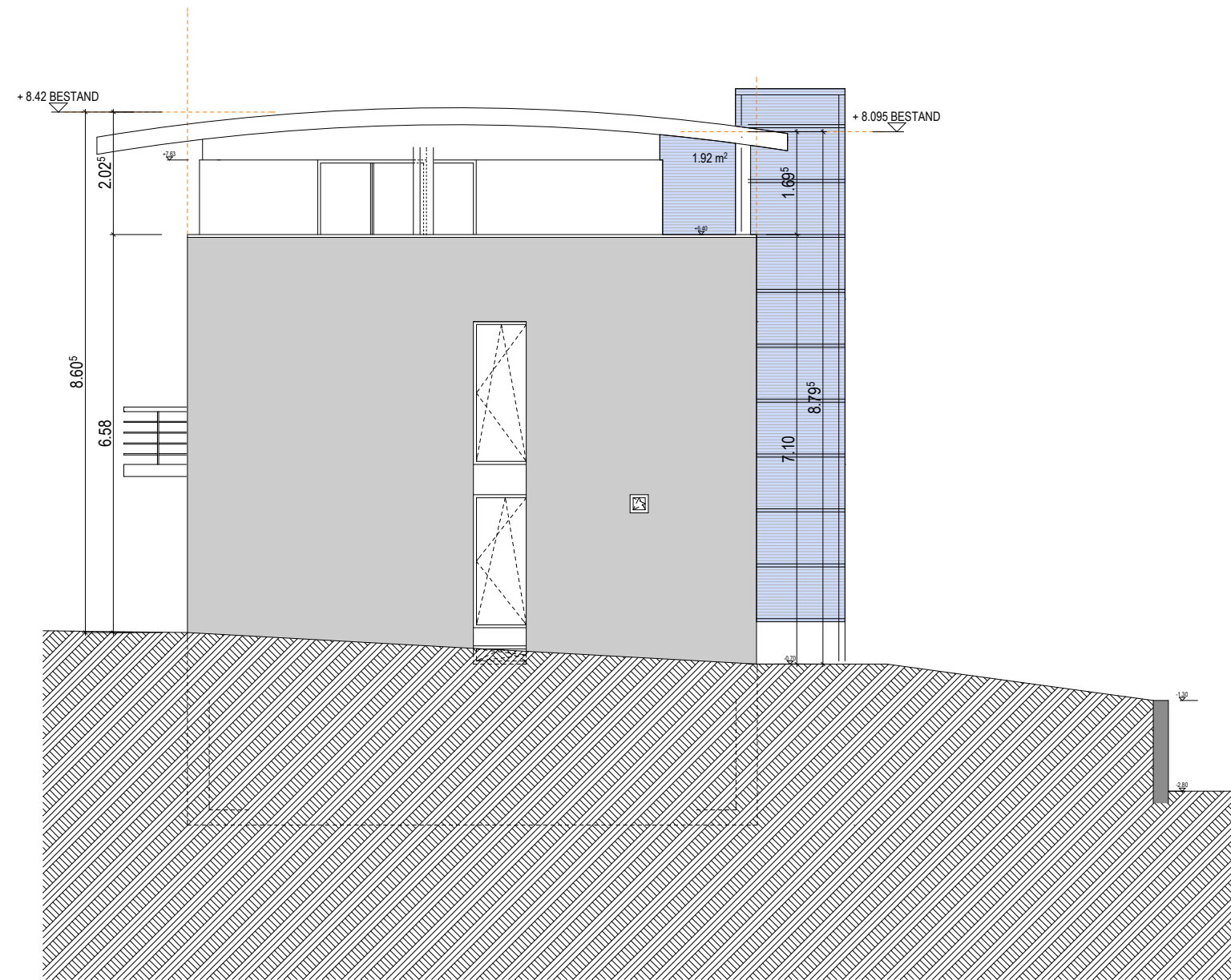
Ansicht Nord
