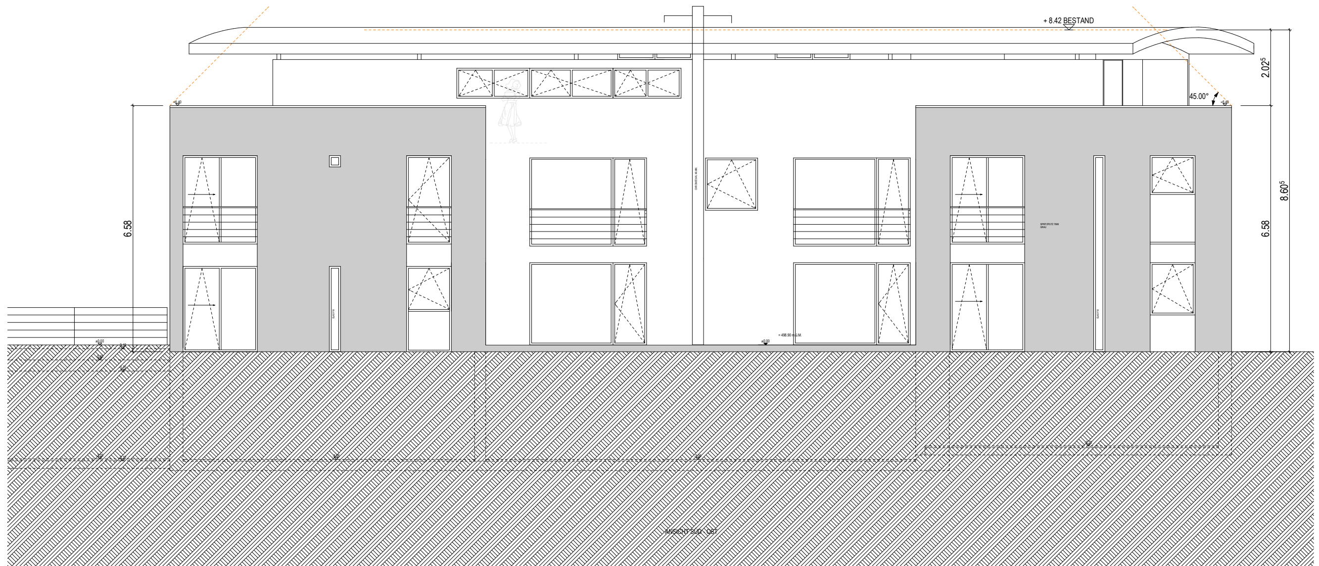
Ansicht Ost
